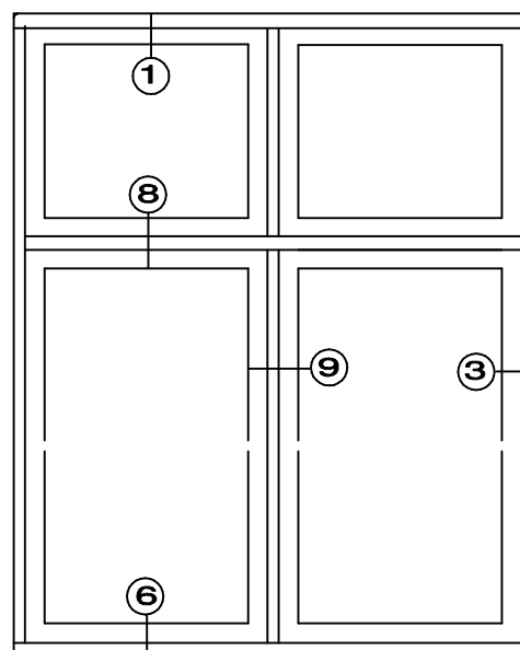
4-Luftfönster med tvärpost
